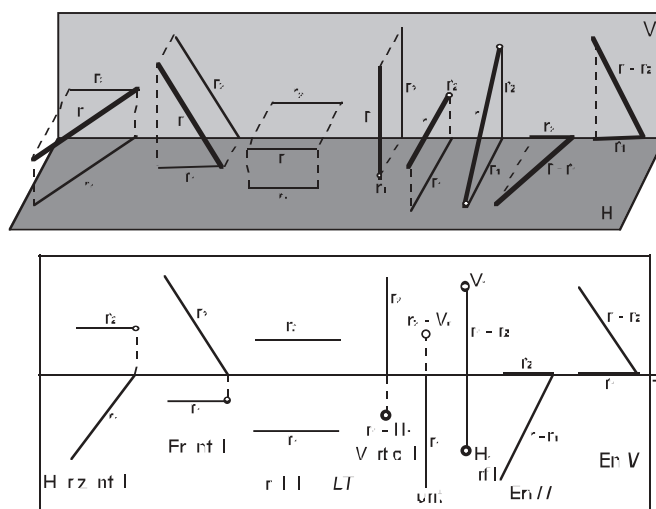
Posiciones relativas de la recta en el espacio.
