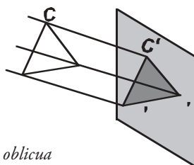
Proyección cilíndrica ortogonal
