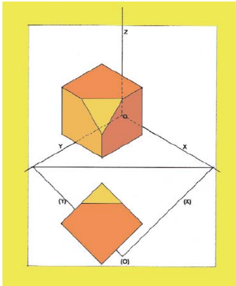
Perspectiva isométrica de un cubo que tiene uno de sus vértices cortado por un plano inclinado 45°.
